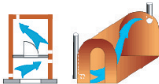
Ventilation croisée en diagonale
